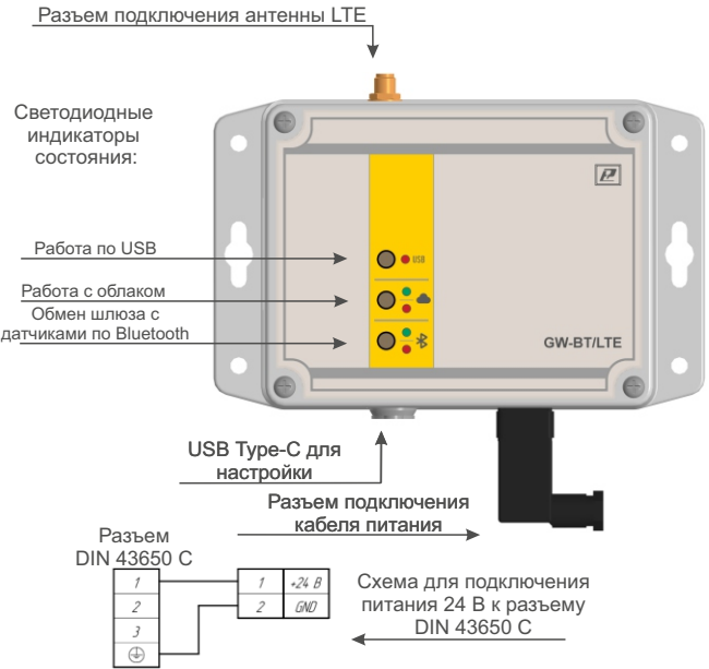
Рисунок 1 - Внешний вид шлюза и схема подключения разъема питания
